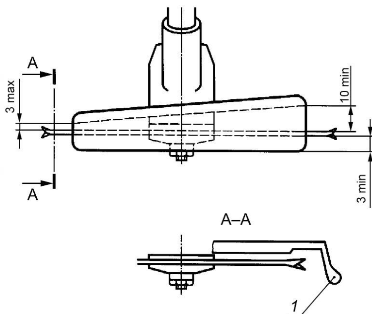
Рисунок 2 — Осевой зазор
