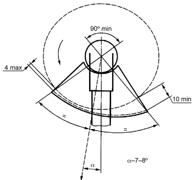
Рисунок 1 — Радиальные зазоры
