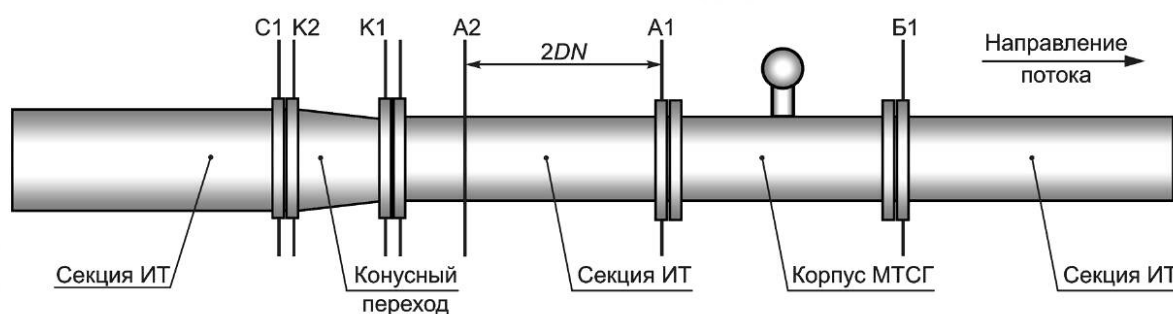
A1, A2, A3, B1, C1 — сечения ИТ; K1, K2 — конусные переходы
