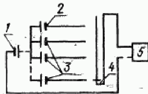
1—вспомогательный Н. Э.; 2—об- разцовый Н. Э.; 3—поверяемый Н. Э.; 4—коммутатор Н. Э.; 5—прибор для определения э.д.с.
