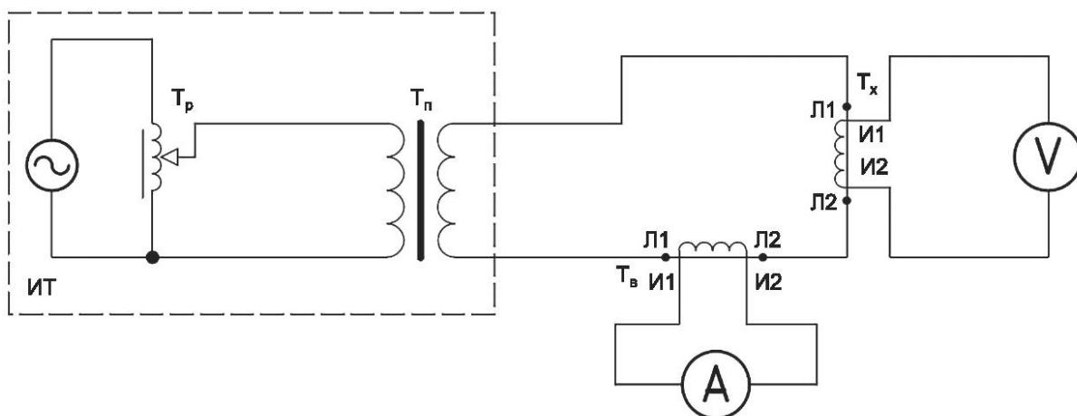
Рисунок Б.1 — Схема размагничивания трансформатора первым способом
