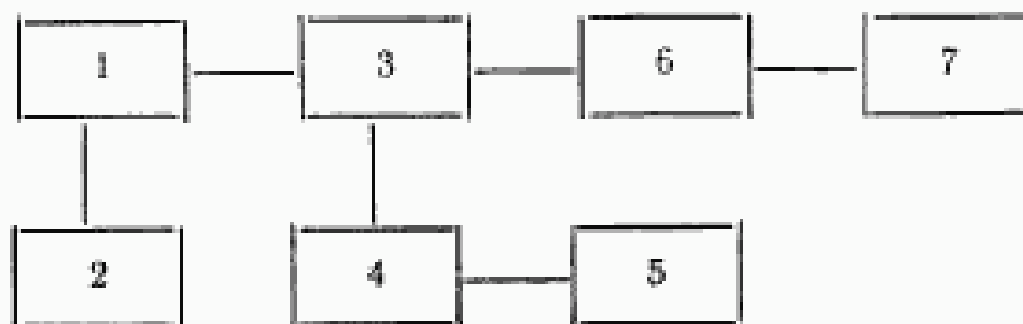
1—измерительный генератор сигналов; 2—импульсный генератор; 3—направленный ответвитель; 4—детекторная секция; 5—осциллограф; 6—измерительный аттенюатор; 7—поверяемый приемник
