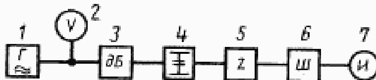
1—генератор; 2—вольтметр; 3—магазин затуханий; 4—согласующее звено; 5—эквивалент микрофона; 6—электрическая часть шумомера; 7—измерительный прибор шумомера
