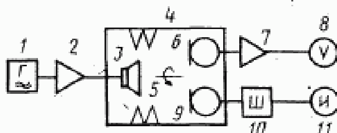
1—генератор; 2—усилитель мощности; 3—громкоговоритель; 4—заклюшенная камера; 5—координатное устройство; 6—образцовый микрофон; 7—микрофонный усилитель; 8—вольтметр; 9—микрофон шумомера; 10—электрическая часть шумомера; 11—измерительный прибор шумомера
