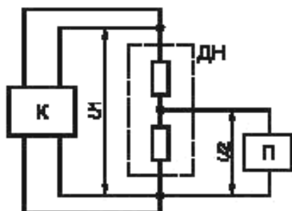
Схема измерения калибратором
