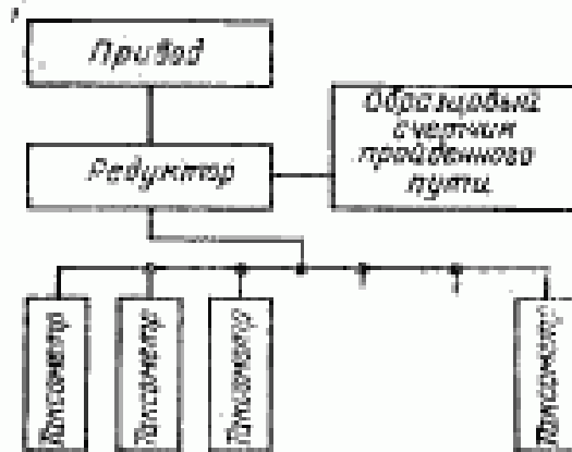
Структурная схема установки для поверки таксометров
