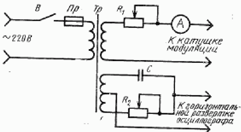
B —выключатель; Pr —предохранитель; R 1 —регулируемый резистор; R 2 —резистор регулировки фазы; C —конденсатор; Tr —трансформатор
