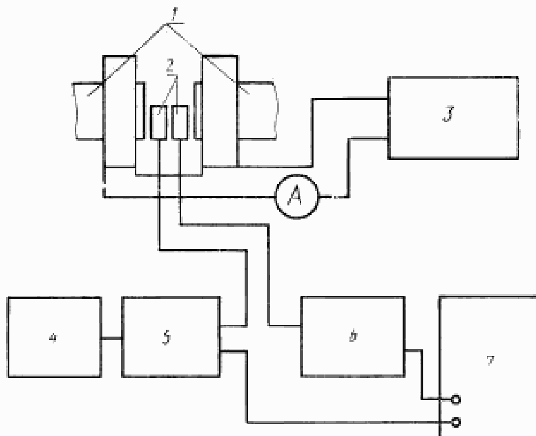
1—полосные наконечники; 2—первичные измерительные преобразователи; 3—источник модулирующего напряжения и фазовращатель; 4—частотомер; 5—образцовый измеритель магнитной индукции; 6—поверяемый тесламетр; 7—двухлучевой осциллограф
