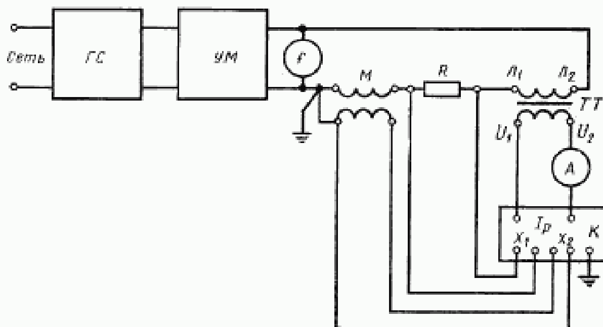
ГС—низкочастотный измерительный генератор сигналов; УМ—усилитель мощности; f—частотомер; К—компенсатор; R—магазин сопротивлений; M—магазин взаимной индуктивности; ТТ—трансформатор тока; А—амперметр.
