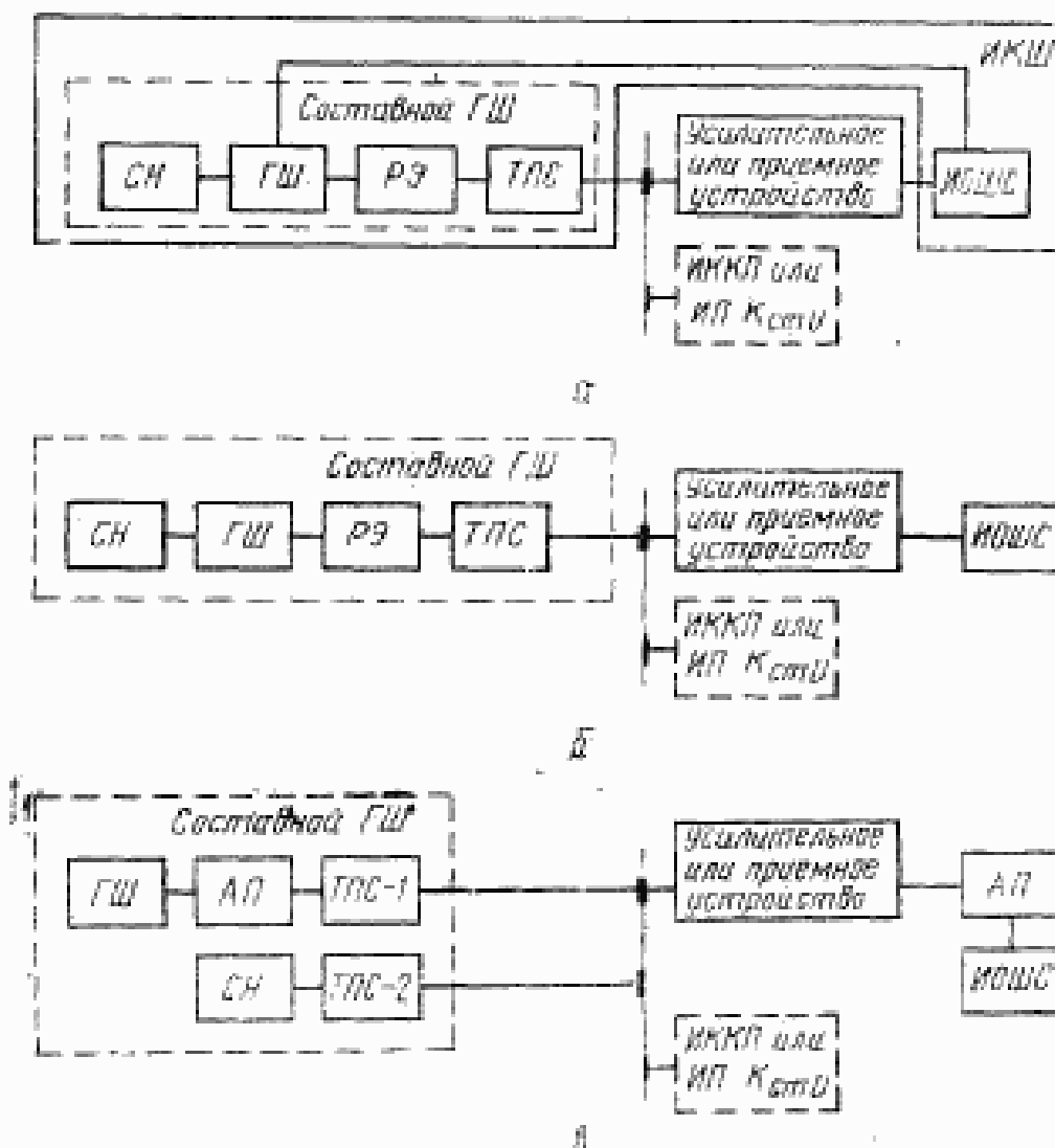
а—схема стенда для измерения коэффициента шума с использованием промодулированного генератора шума (ГШ); б—то же, методом двух отсчетов; в—схема стенда для предельных измерений с использованием аттестованного поляризованного аттенюатора (АП)
