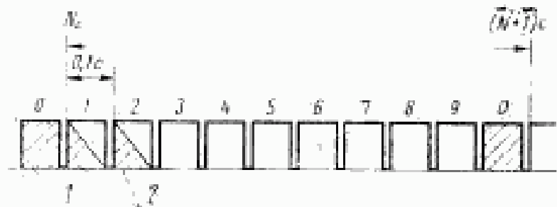
1—секундный маркер; 2—информационные сигналы
