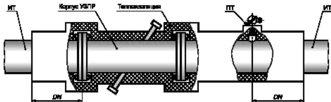
Рисунок 6 — Пример теплоизоляции корпуса УЗПР и участков ИТ
