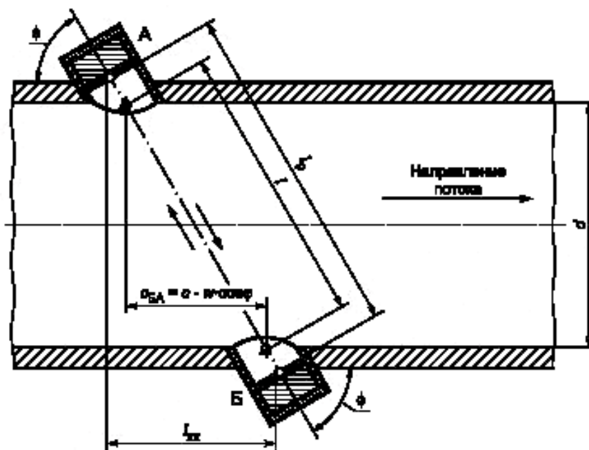
Рисунок 1 — Схема одноканального УЗПР с ПЗА, размещенными в стенке его корпуса
