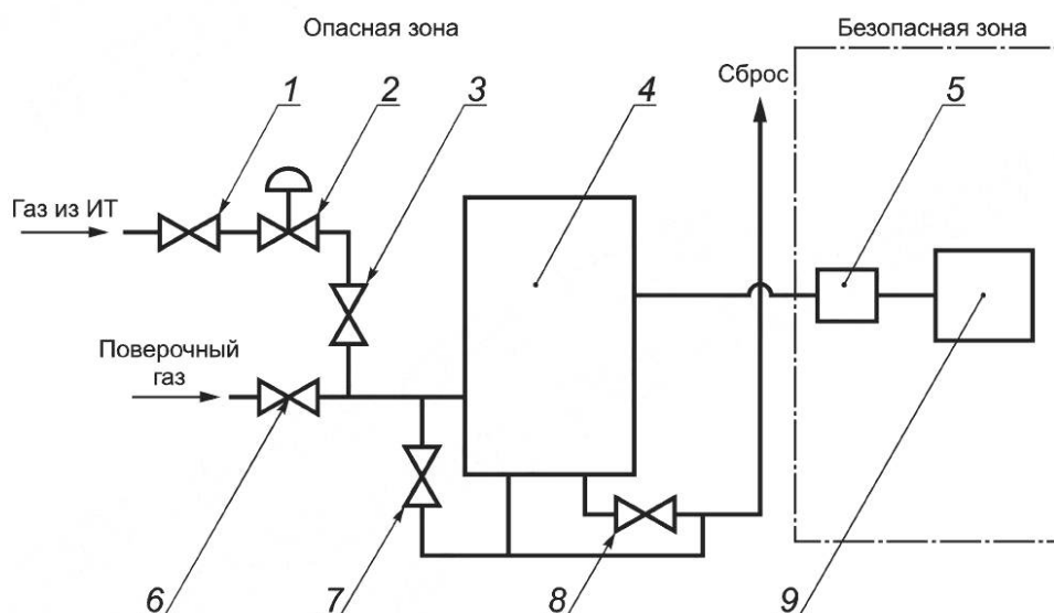
Рисунок 7 — Типовая схема монтажа потокового плотномера для измерения плотности газа при стандартных условиях
