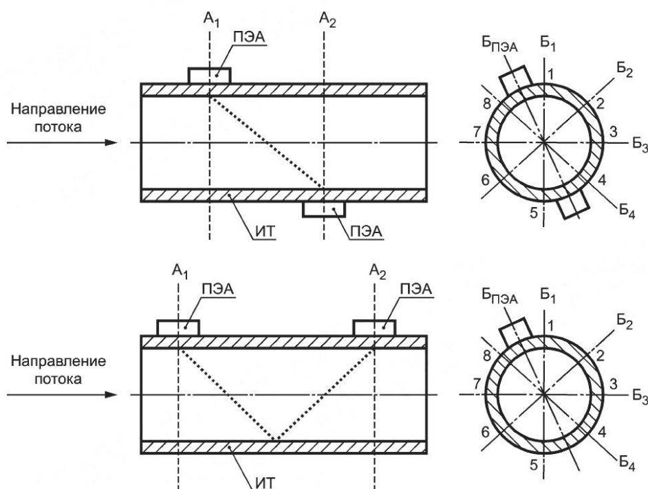
Рисунок 4 — Сечения ИТ и диаметрально-направленные измерения, в которых выполняют измерения наружного диаметра ИТ
