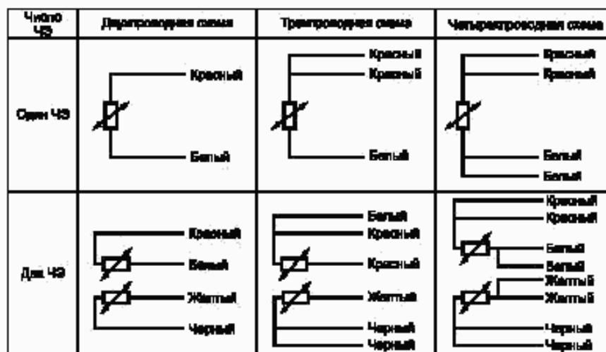
Рисунок 1 — Схемы соединения внутренних проводов
