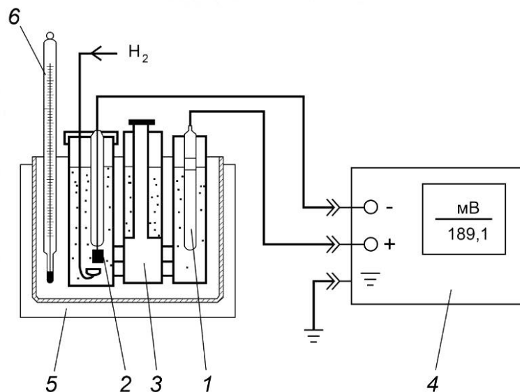
Схема установки для определения потенциала эталонного электрода сравнения E_{\text{эт}}
