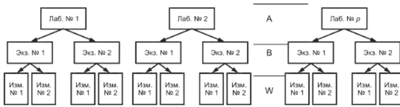
Рисунок А.1 — Схема проведения совместных исследований одновременно с исследованием однородности партии [определение значения аттестуемой характеристики материала CO (двухфакторный план эксперимента)]
