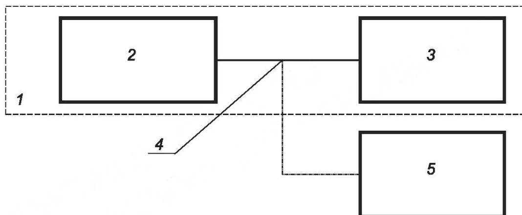
Рисунок 6 — Блок-схема установки для сличения ИОП с РЭОП
