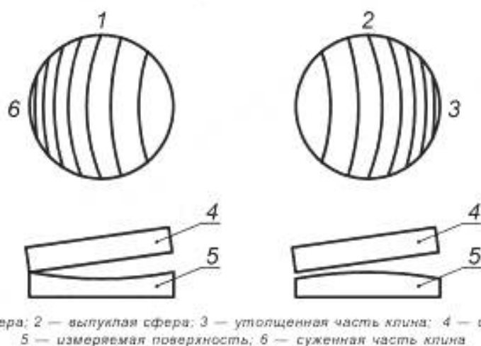
Рисунок 5 — Смещение полос в случае вогнутой и выпуклой поверхностей соответственно
