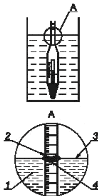
1 — жидкость; 2 — точка записи показаний; 3 — горизонтальная поверхность; 4 — мениск
