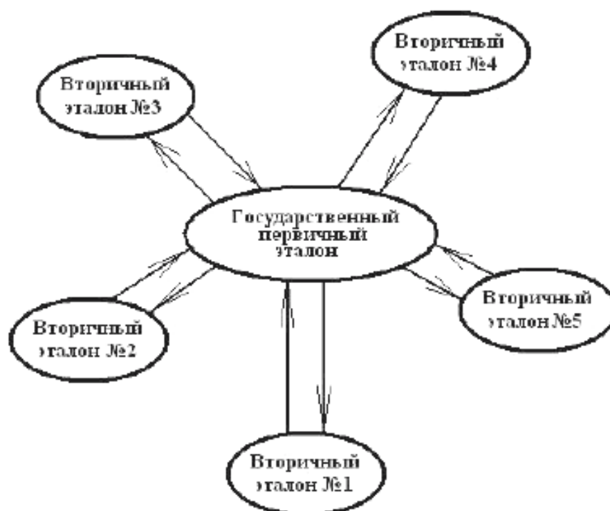
Рисунок 2 – Звездная схема процедуры сличений
