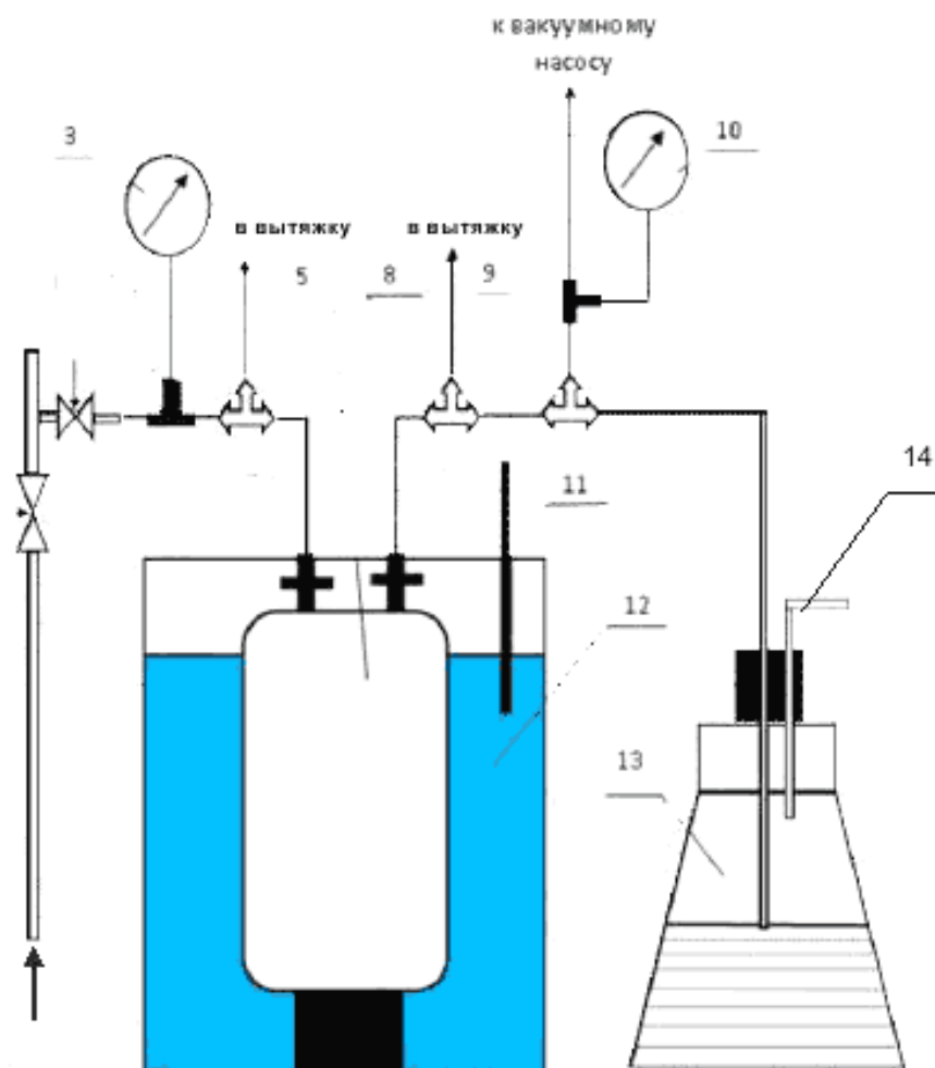
1 – кран; 2 – Т-образный тройник; 3 – манометр; 4, 6 – клапаны; 5 – calorиметрическая бомба; 7, 8, 9 – краны соединительные трехходовые; 10 – вакуумметр; 11 – термометр; 12 – термостат; 13 – контрольная склянка; 14 – капиллярная трубка
