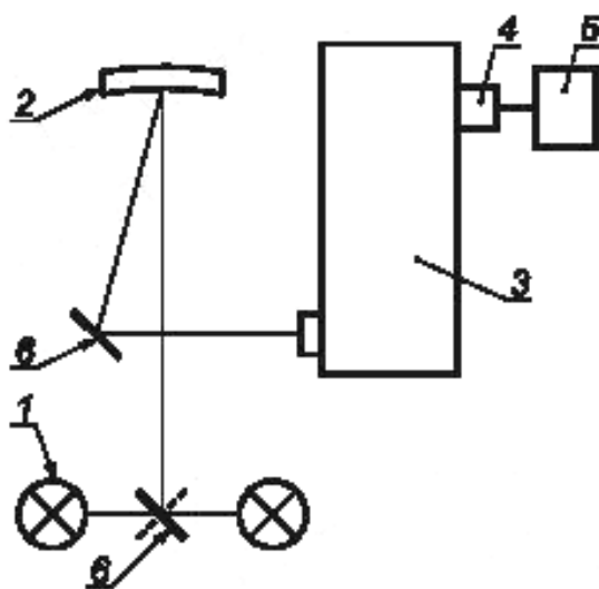
Рисунок 1 — Блок-схема установки для измерения СПЭО
