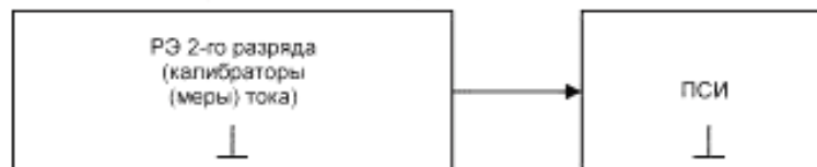
Рисунок 6 — Схема соединения приборов при поверке РСИ в диапазоне токов от 1 \cdot 10^{-15} до 1 \cdot 10^{-9} А на РЭ 2-го разряда, в качестве которых используют калибраторы (меры) тока
