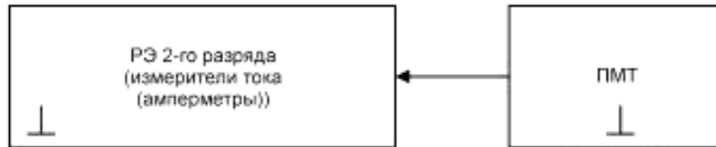
Рисунок 5 — Схема соединения приборов при поверке РСИ в диапазоне токов от 1 \cdot 10^{-15} до 1 \cdot 10^{-9} А на РЭ 2-го разряда, в качестве которых используют измерители тока (амперметры)
