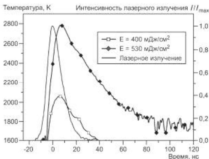
Рисунок А.4 — Динамика изменения температуры ртути при больших плотностях энергии лазерного излучения
