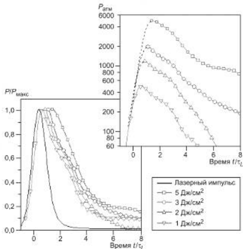
Рисунок А.8 — Динамика изменения давления в алюминиевом образце при больших плотностях энергии лазерного излучения
