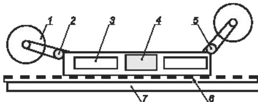
1 — шнек с резцами; 2 — поворотный редуктор; 3 — отделение редуктора; 4 — распределительное устройство; 5 — электродвигатель привода шнека; 6 — расположение реечной передачи; 7 — забойный скребковый конвейер
