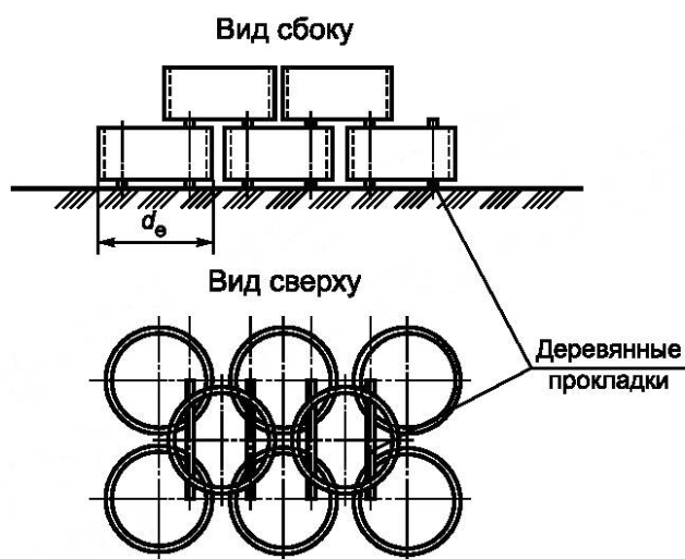
Рисунок 1 — Складирование стеновых колец колодцев
