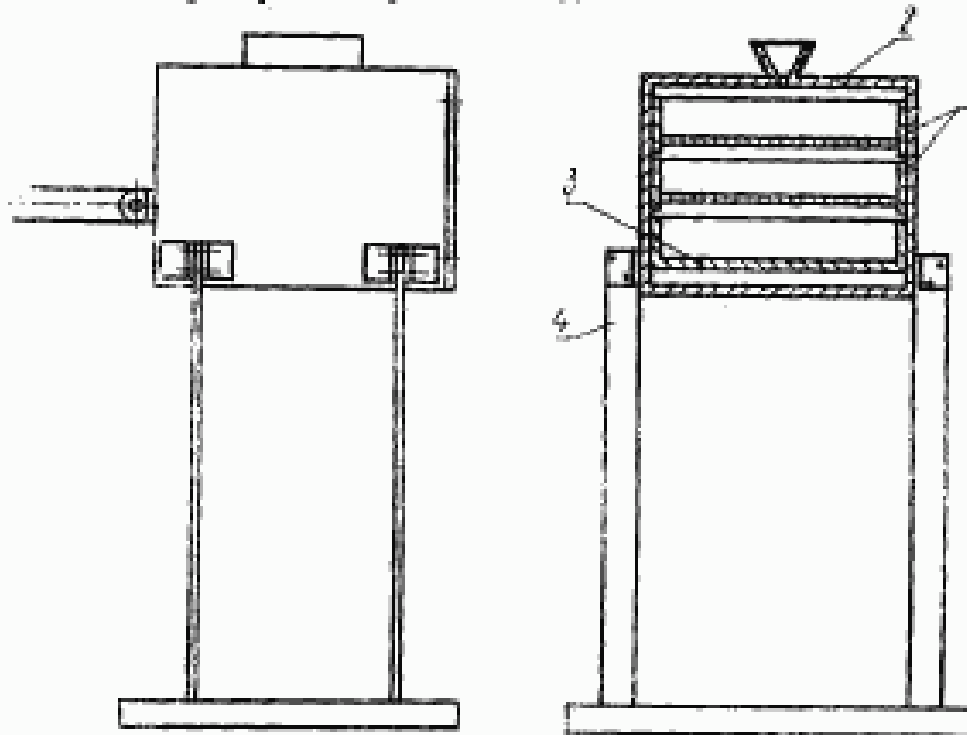
Прибор для определения фракционного состава
