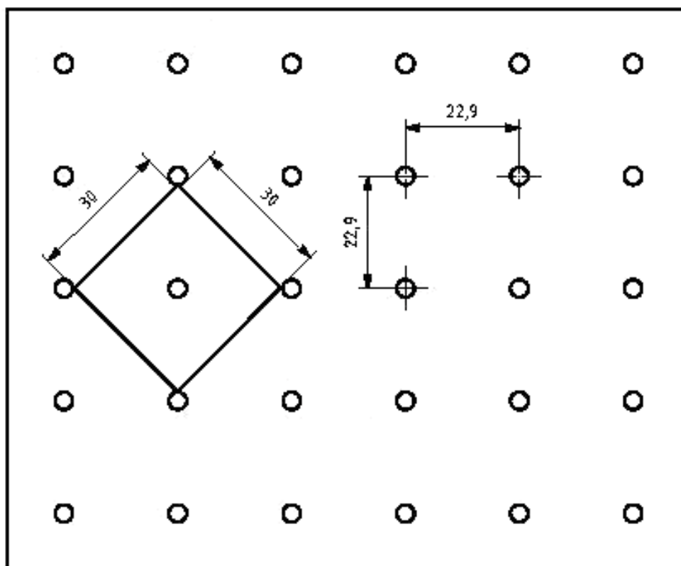
Рисунок 11 — Пример рисунка перфорации
