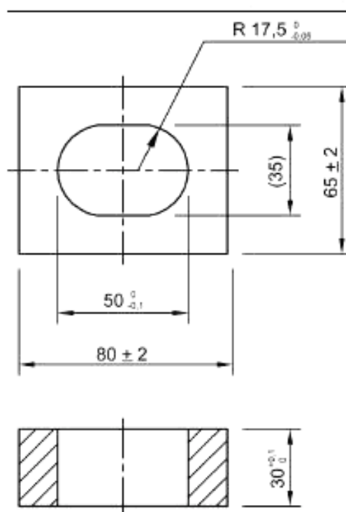
Рисунок 18 — Испытательный шаблон А
