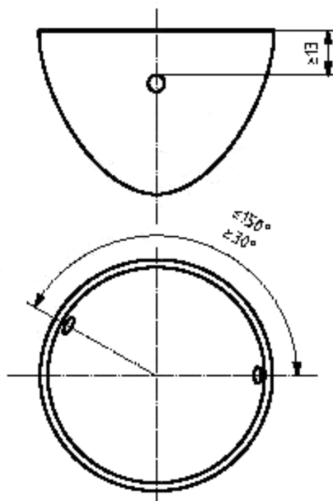
б) Расположение отверстий
