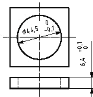
Рисунок 20 — Испытательный шаблон С
