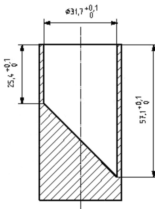
Рисунок 17 — Цилиндр для мелких деталей
