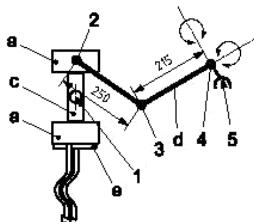
b) испытательный груз для самокатов, предназначенных для детей массой не более 20 кг
