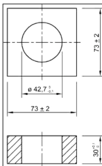
Рисунок 18 — Испытательный шаблон А
