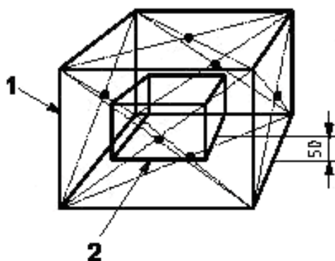
1 — измерительный куб; 2 — контрольный куб
