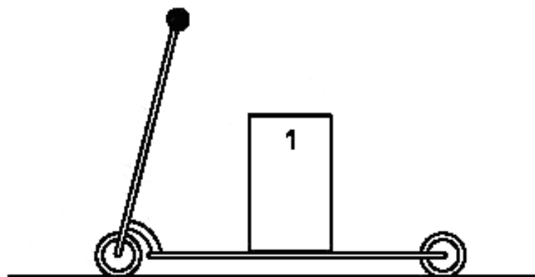
1 — испытательный груз
