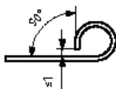
a) Завернутая кромка
