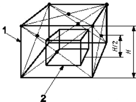
1 — измерительный куб; 2 — контрольный куб
