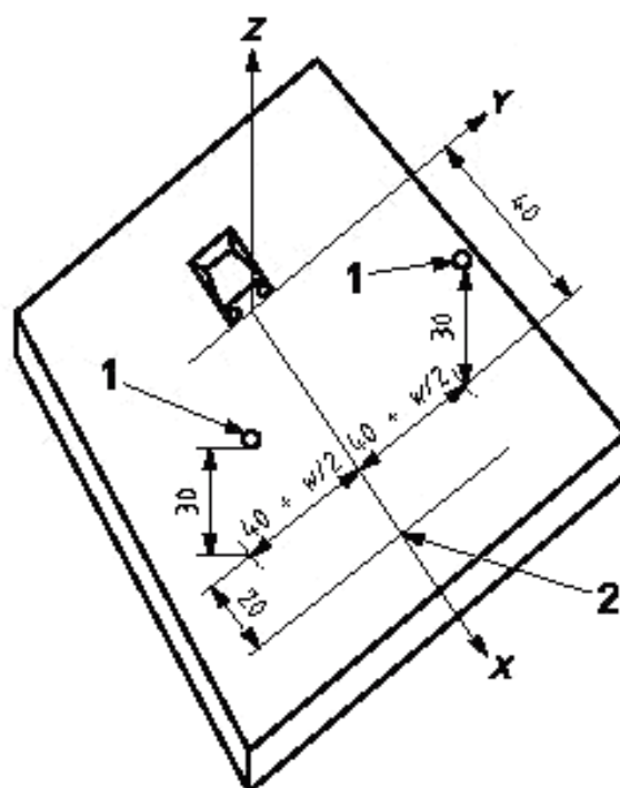
1 — микрофон; 2 — конец измерения; W — ширина игрушки
