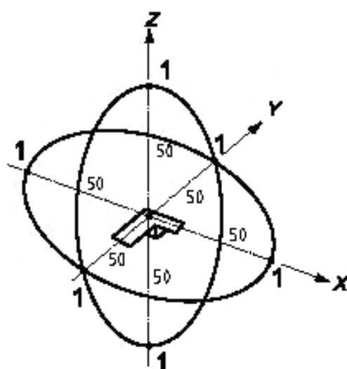
1 — микрофон
