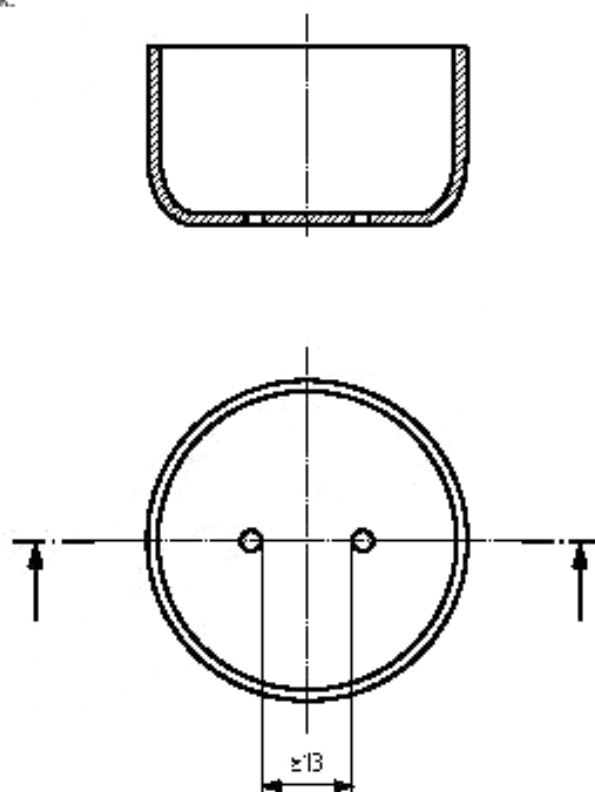
а) Отверстия в основании чаши
