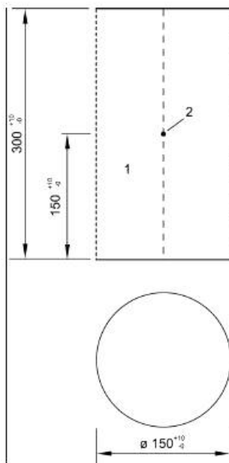
1 — масса, 50 кг или 100 кг; 2 — центр тяжести
