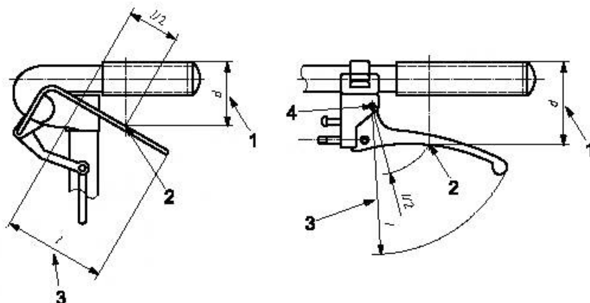
1 — размер рычага ручного тормоза; d; 2 — середина рычага; 3 — длина рычага; 4 — ось опоры рычага
