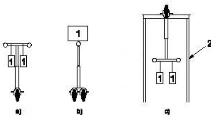
1 — испытательный груз, 2 — подиум
