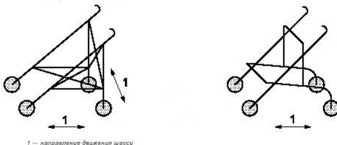
Рисунок 13 — Детские колесные кресла, подпадающие под 4.12.1 б)
