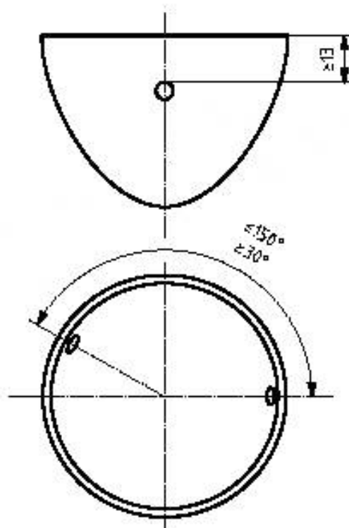
б) Расположение отверстий
