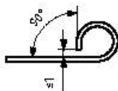
a) Завернутая кромка
