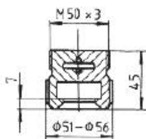
с) Деталь В – устройство сопряжения резьбового соединения с деталью С
