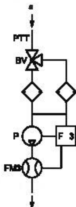
Рисунок 20 – Система пробоотбора частиц
