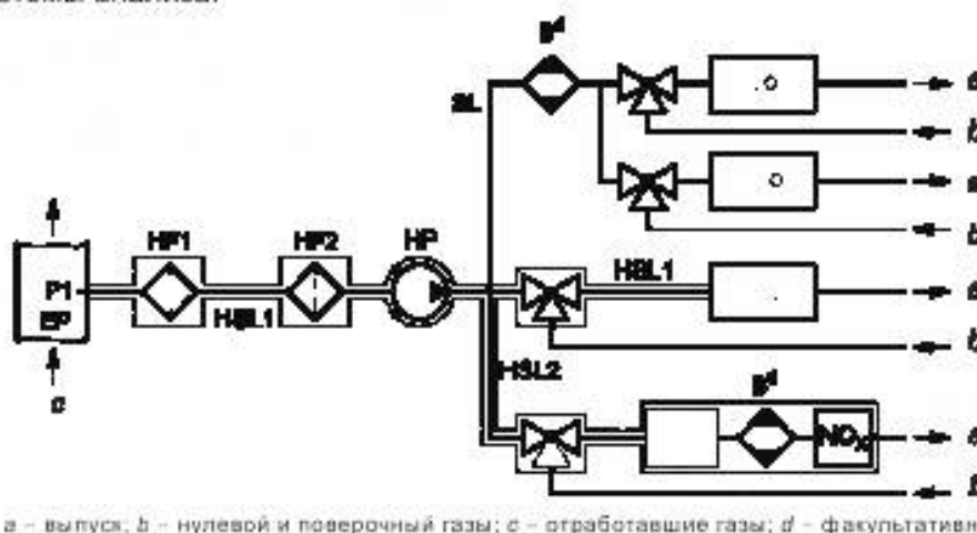
Рисунок 3 – Блок-схема системы анализа неразбавленных отработавших газов на содержание CO, CO 2 , NO x , HC и O 2
