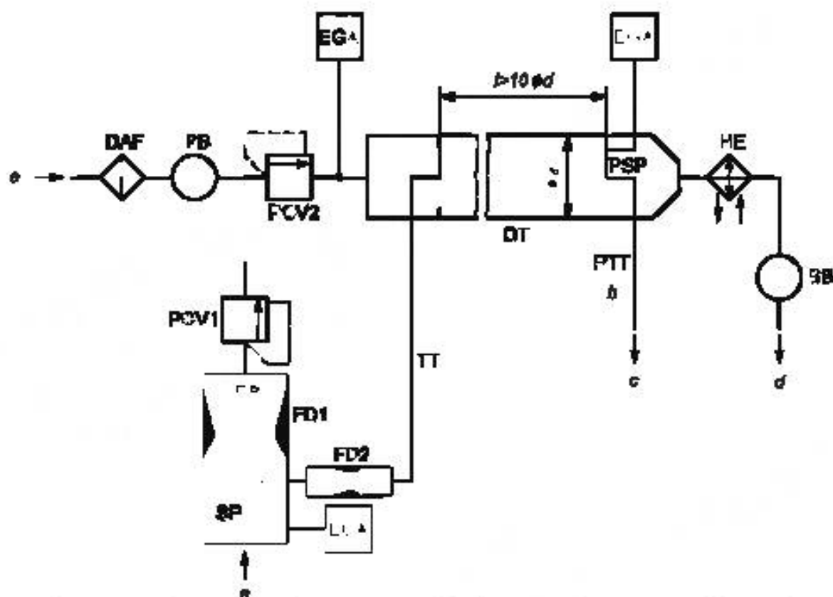
а – отработавшие газы; б – см. рисунок 20; в – в систему пробоотбора частиц; д – выпуск; е – разбавляющий воздух. Рисунок 15 – Частичнопоточная система разбавления с двумя трубками Вентури или с двумя отверстиями, измерением концентрации и фракционным пробоотбором
