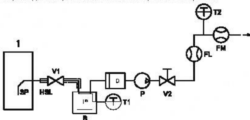
Рисунок 8 – Блок-схема системы анализа на метанол
