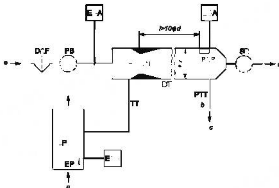
а – отработавшие газы, б – см. рисунок 20; с – в систему пробоотбора частиц; d – выпуск; e – разбавляющий воздух Рисунок 14 – Частичнопоточная система разбавления с одной трубкой Вентури, измерением концентрации и фракционным пробоотбором
