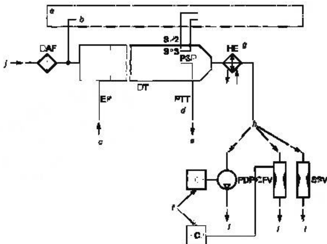
а – анализатор, см рисунок 4; б – фон; с – отработавшие газы; d – см. рисунок 20; е – в систему пробоотбора, см. рисунок 20, или в DDS, см. рисунок 21; f – при использовании EFC; g – факультативно; h – или-или; i – выпуск; j – разбавляющий воздух
