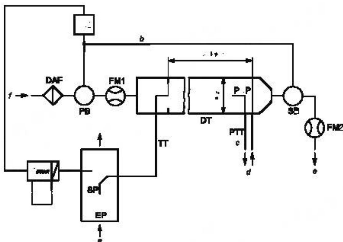
а – отработавшие газы; б – в PB или SB; с – см. рисунок 20; d – в систему пробоотбора частиц; e – выпуск; f – разбавляющий воздух
