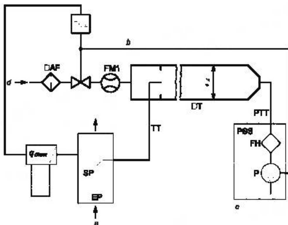
а – отработавшие газы; б – в Р (PSS) (факультативно); с – см. рисунок 20; d – разбавляющий воздух Рисунок 17 – Частичнопоточная система разбавления с измерением расхода и общим пробоотбором
