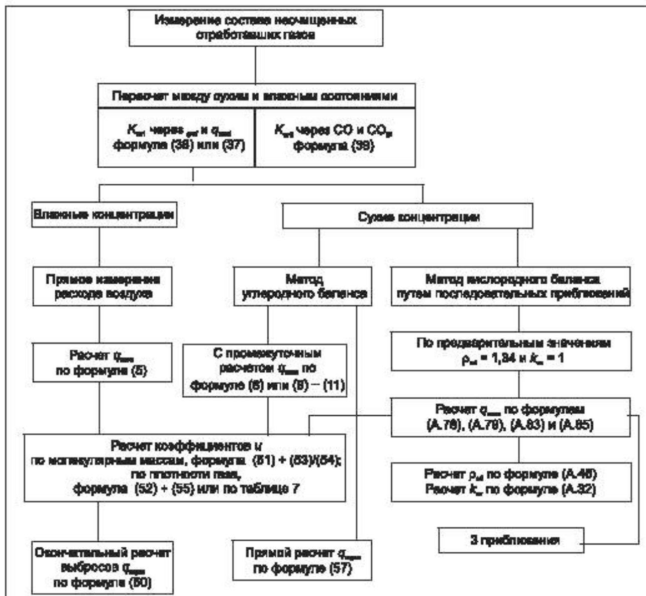
Рисунок 2 – Измерение состава неразбавленных отработавших газов
