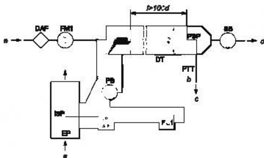
а – отработавшие газы; б – см. рисунок 20; с – в систему пробоотбора частиц; d – выпуск; e – разбавляющий воздух. Рисунок 11 – Частичнопоточная система разбавления с изокINETическим пробоотборником и фракционным пробоотбором (управление нагнетателем на выпуске PB)
