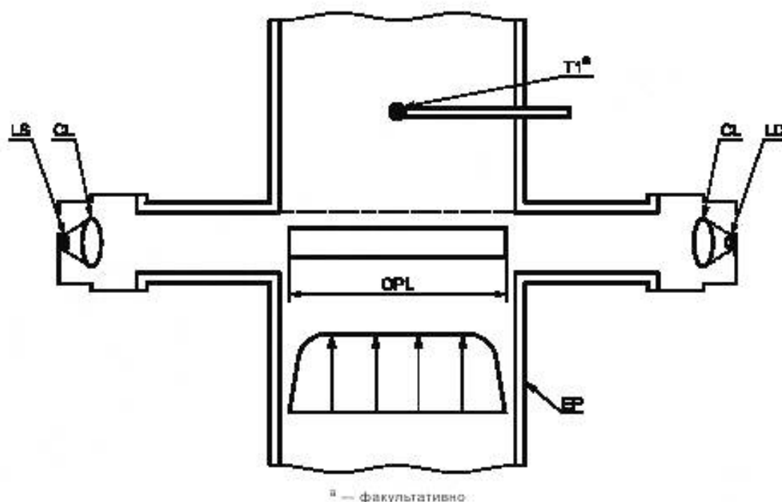
Рисунок 1 — Полнопоточный оптический дымомер
