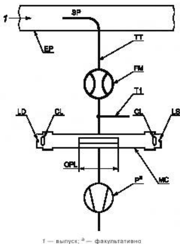
Рисунок 2 — Частично поточный оптический дымомер
