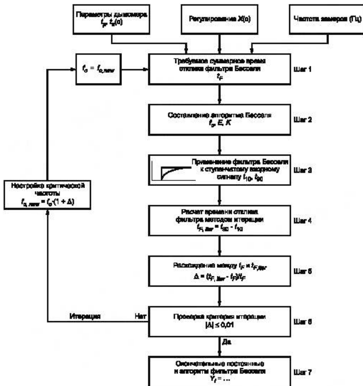
Рисунок D.2 — Схема итерации по алгоритму Бесселя
