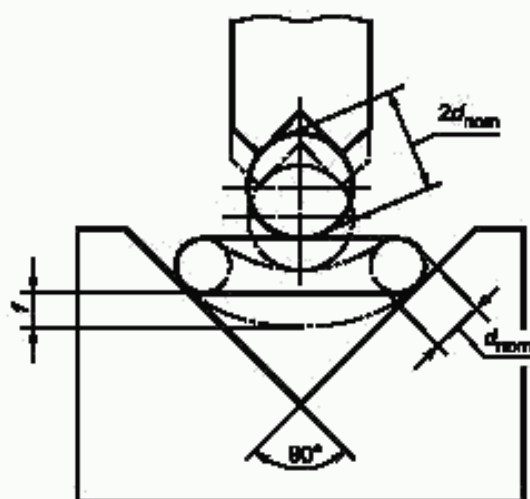
Рисунок 1 — Прогиб f
