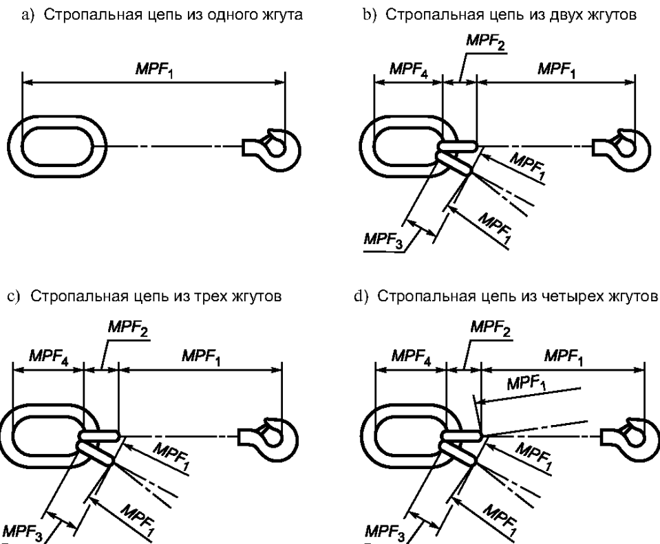
Рисунок 6 — Испытательные участки стропальных цепей
