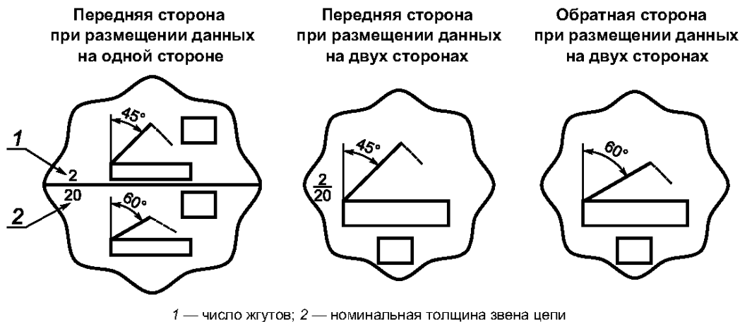
Рисунок D.2 — Ярлыки для маркировки стропальных цепей из нескольких жгутов
