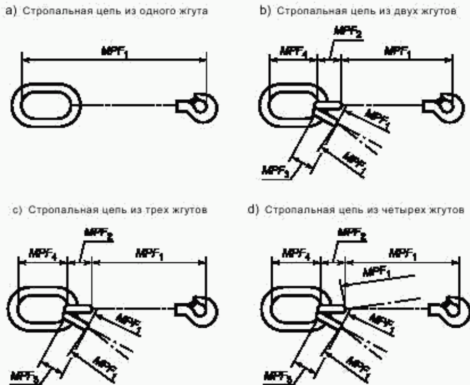
Рисунок 5 — Испытательные участки стропальных цепей
