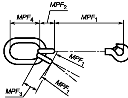
б) Стропальная цепь из двух жгутов
