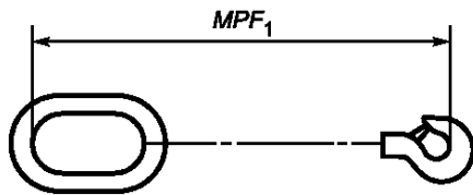
а) Стропальная цепь из одного жгута
