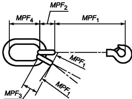
Рисунок 5 — Испытательные участки стропальных цепей
