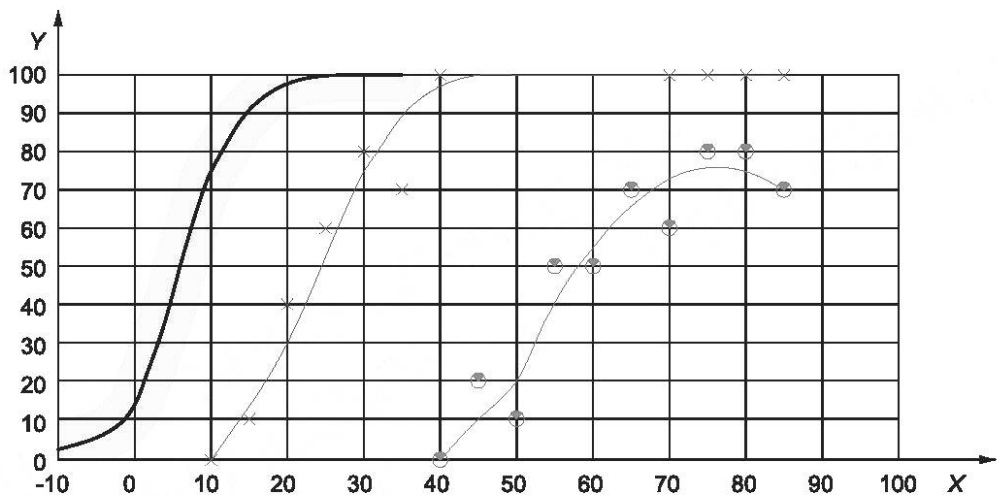
Рисунок С.2 — Пример речевой аудиограммы для речевого материала в форме однословных слов
