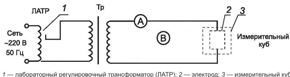
Рисунок 10 — Измерительная схема
