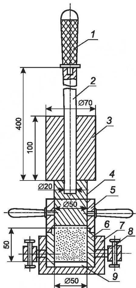
1 — рукоятка; 2 — направляющий стержень; 3 — гиря; 4 — плунжер; 5 — направляющий насадный цилиндр; 6 — разъемный цилиндр; 7 — подстаканник; 8 — закрепляющие винты; 9 — металлическая пластинка
