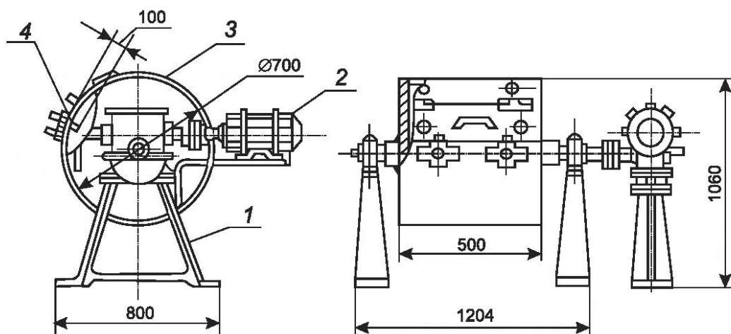
1 — станина; 2 — двигатель; 3 — барабан; 4 — полка барабана
