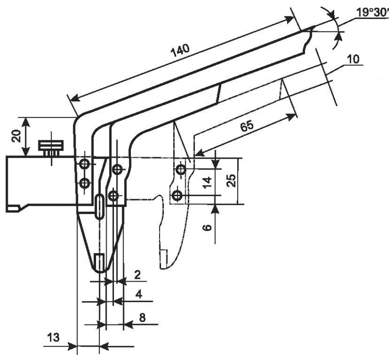
Рисунок 3 — Передвижной шаблон
