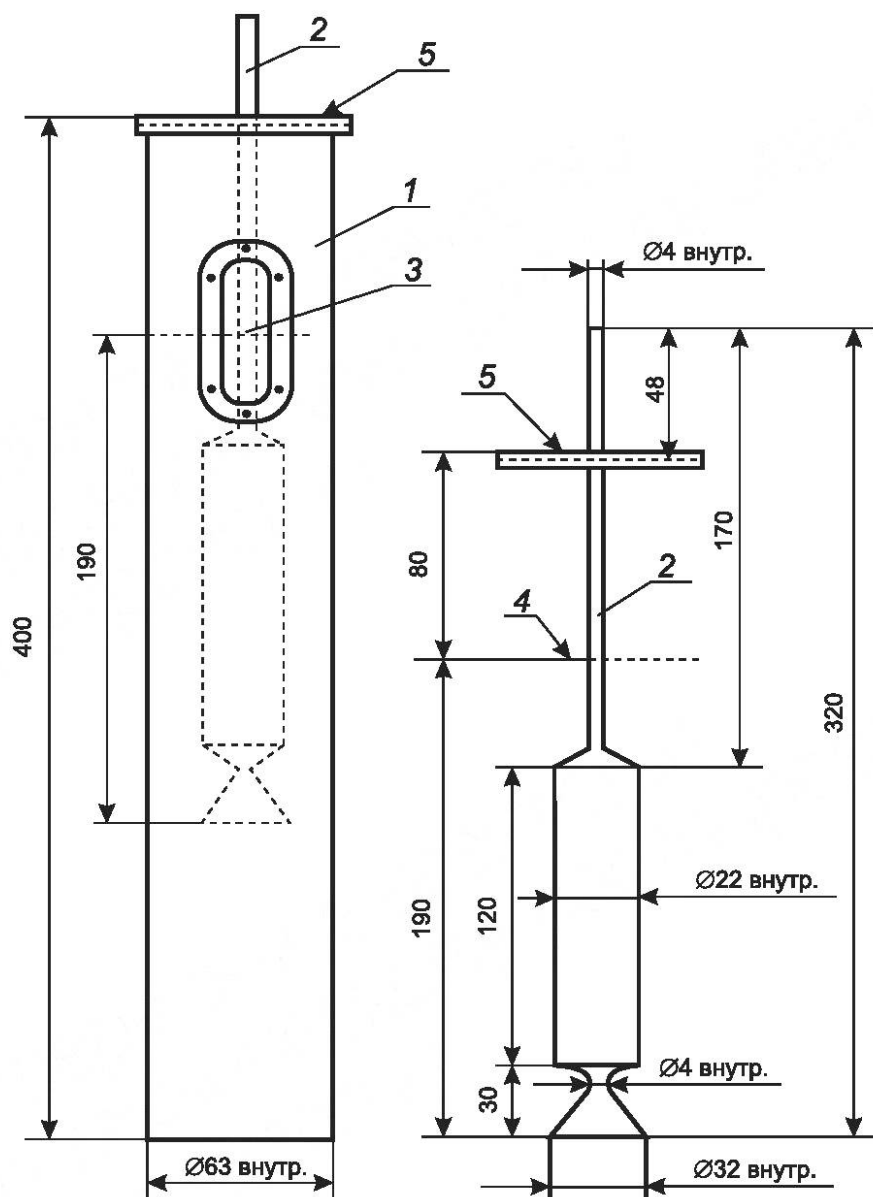
1 — цилиндр; 2 — пипетка; 3 — метка на цилиндре (1000 мл); 4 — уровень суспензии в цилиндре; 5 — опорная крышка пипетки
