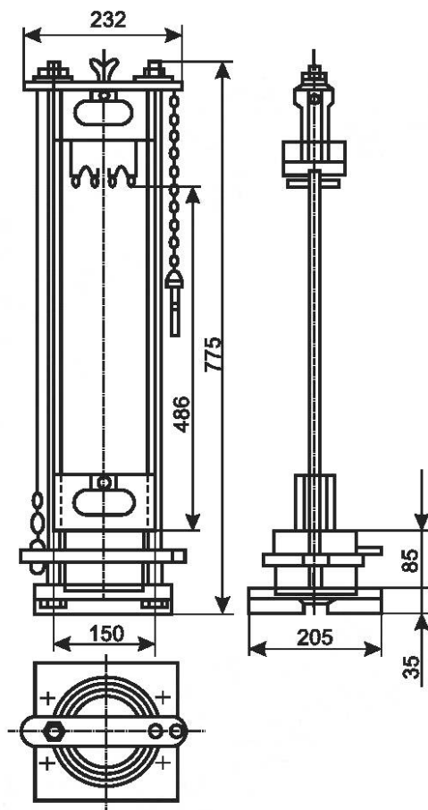
Рисунок 11 — Копер ПМ
