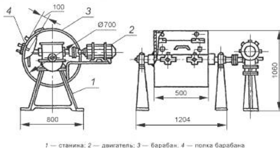
Рисунок 6 — Полочный барабан
