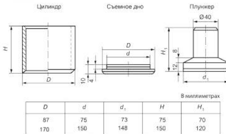
Рисунок 4 — Цилиндры стальные
