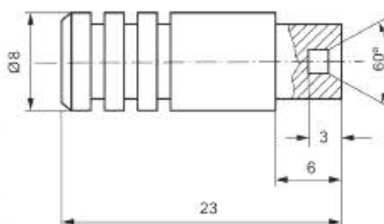
Рисунок 13 — Репер для испытаний
