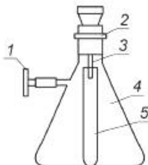
1 — водоструйный насос; 2 — резиновая пробка; 3 — воронка с фильтром Шотта; 4 — склянка Бунзена, 5 — пробирка для сбора фильтрата
