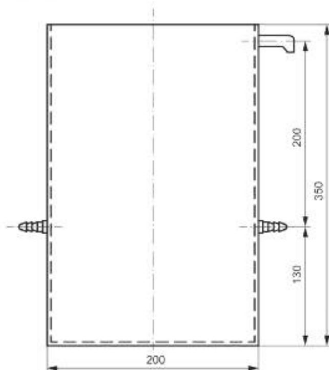
Рисунок 1 — Сосуд для отмучивания
