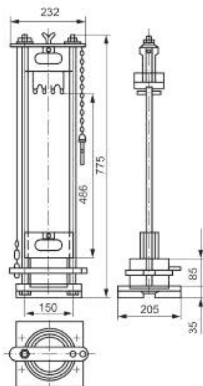
Рисунок 7 — Копер ПМ
