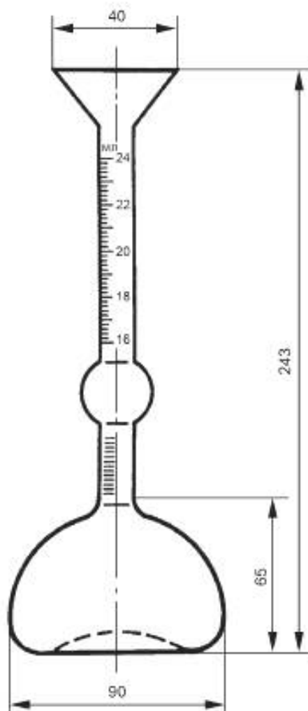
Рисунок 8 — Прибор Ле Шателье
