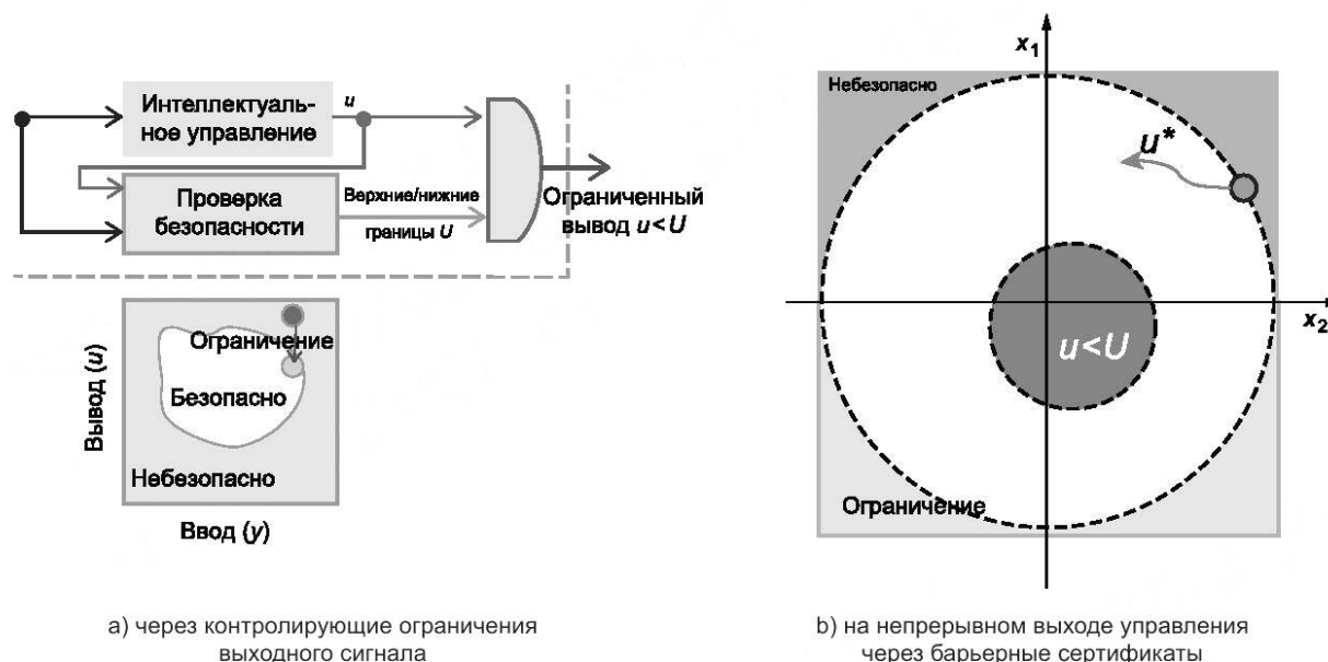
Рисунок 7 — Безопасное применение технологии ИИ для управления
