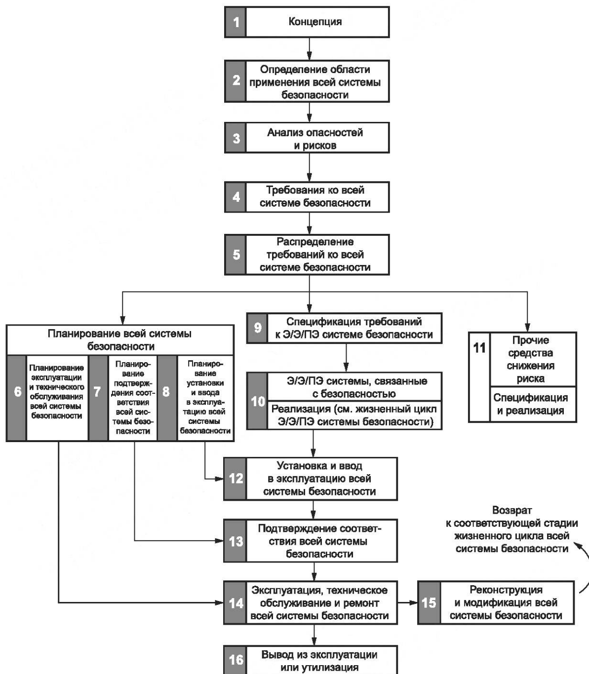
Рисунок 8 — Модель жизненного цикла (ГОСТ Р МЭК 61508-1—2012, рисунок 2)
