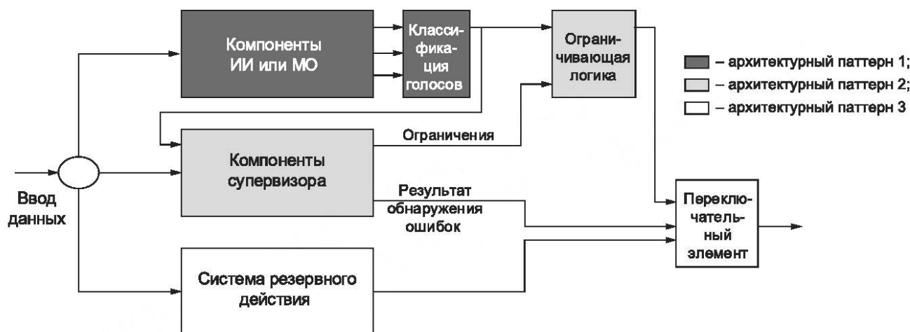
Рисунок 5 — Архитектурные паттерны для систем, использующих компоненты ИИ
