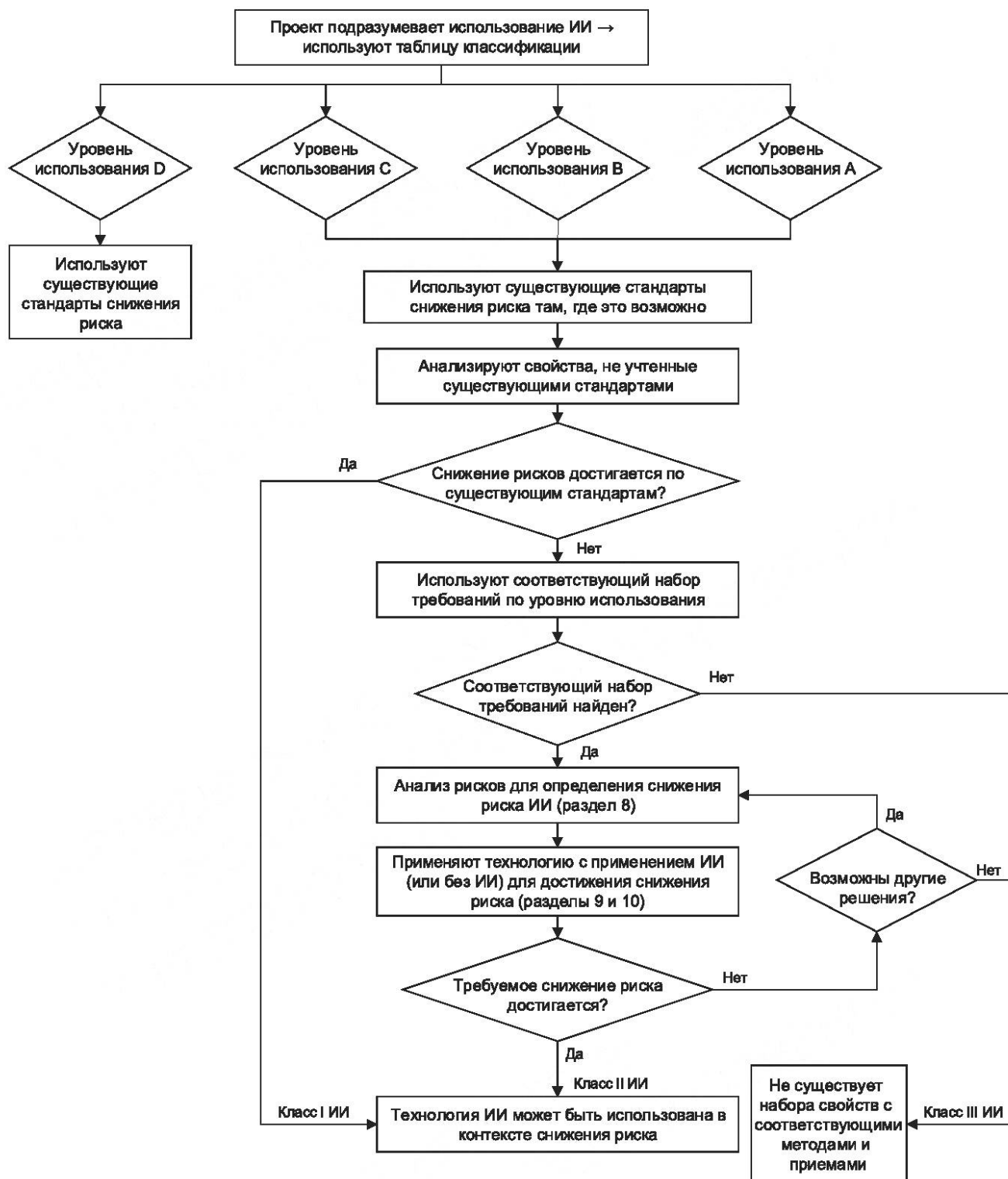
Рисунок 1 — Блок-схема для определения классификации технологий ИИ
