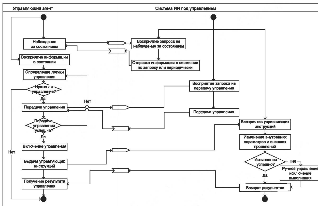
Рисунок 2 — Диаграмма действия процесса управления
