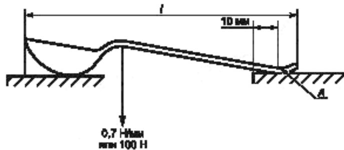
Рисунок 1 — Испытание ложки на прочность
