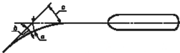
Рисунок D.2 — Определение угла остаточной деформации
