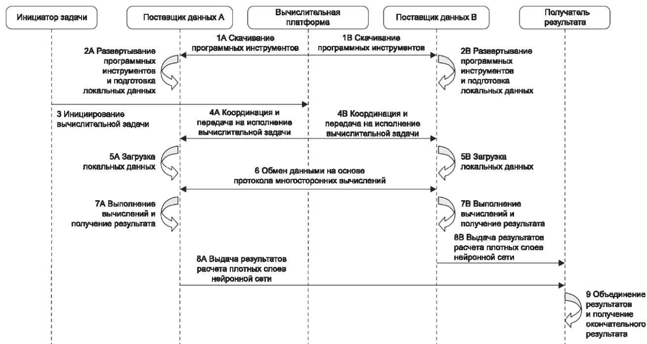
Рисунок 5 — Процедуры обработки федеративной системы МО в децентрализованном режиме
