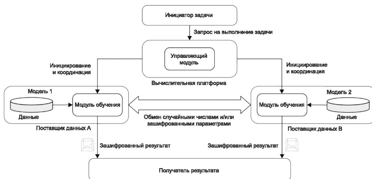
Рисунок 4 — Техническая архитектура федеративной системы МО в децентрализованном режиме
