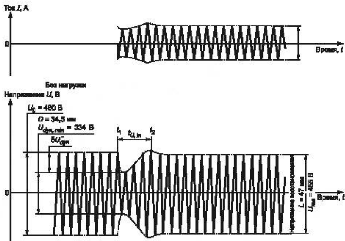
Рисунок А.3 — Переходное напряжение генератора в зависимости от времени при внезапном увеличении нагрузки
