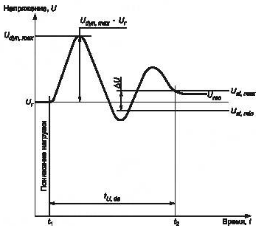
Рисунок А.2 — Характеристика переходного напряжения (понижение нагрузки)
