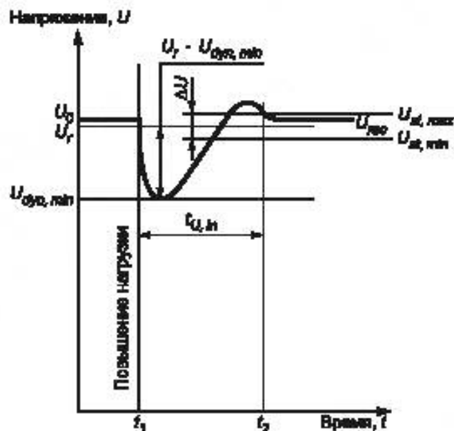
Рисунок А.1 — Характеристика переходного напряжения (повышение нагрузки)
