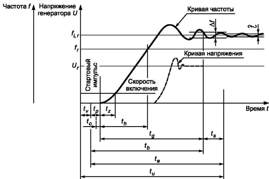
Рисунок 10 — Пусковые характеристики
