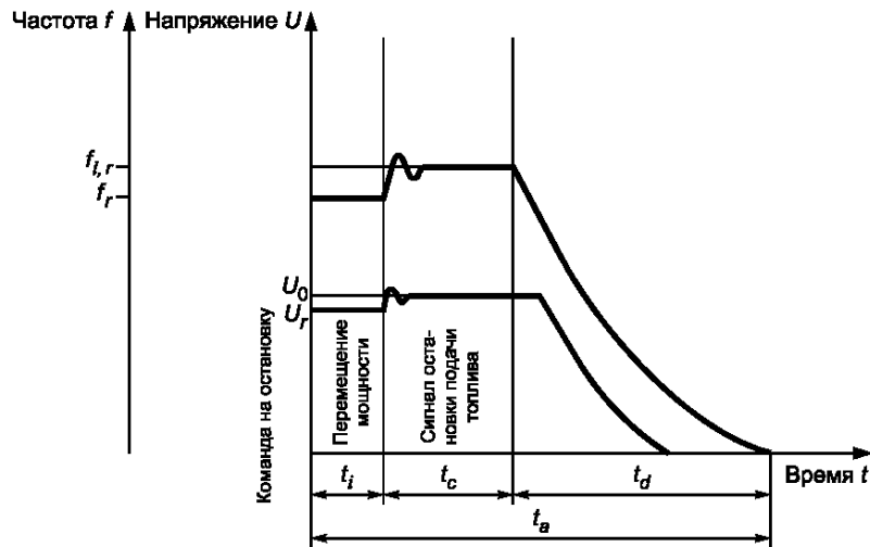
Рисунок 11 — Характеристики остановки
