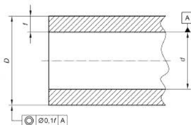
Рисунок 1 — Соосность наружного диаметра трубы
