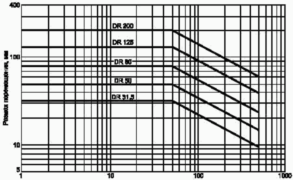
Рисунок 1 — Кривые классов вибрации для вибрации вала
