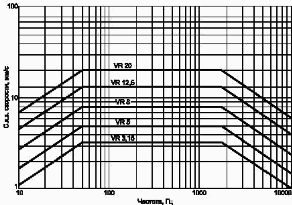
Рисунок 2 — Кривые классов вибрации для вибрации корпуса
