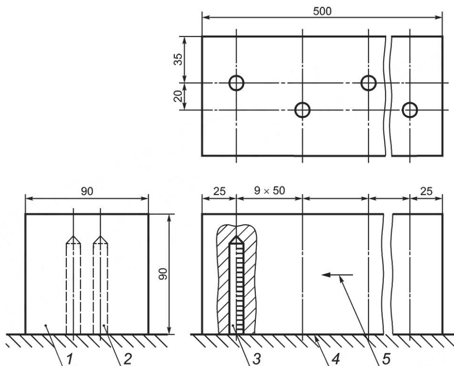
1 — основа; 2 — глухие отверстия; 3 — вставка; 4 — обрабатываемая сторона плиты; 5 — направление подачи
