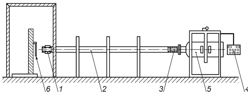
1 — спидометр; 2 — ствольный канал; 3 — летящий предмет; 4 — пульт управления; 5 — сосуд со сжатым воздухом; 6 — испытываемый объект
