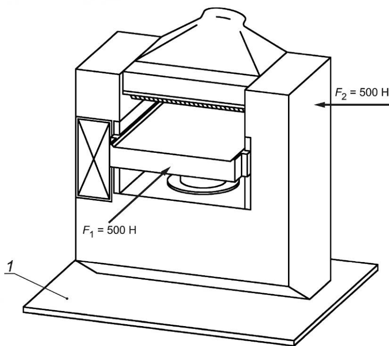
Рисунок В.1 — Испытание на устойчивость передвижных станков
